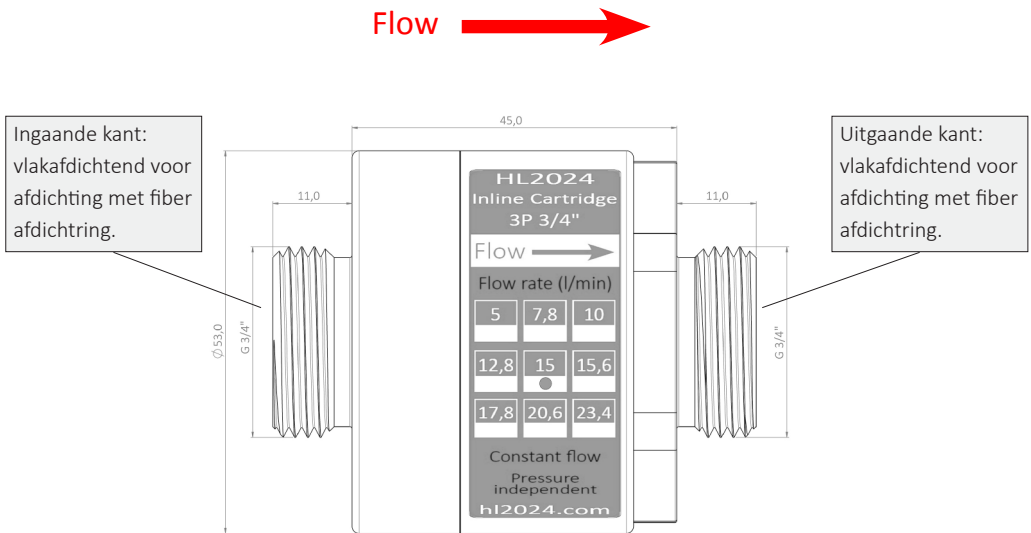
Afbeelding: HL2024 Inline Cartridge 3P 3/4" (afmetingen in mm)
