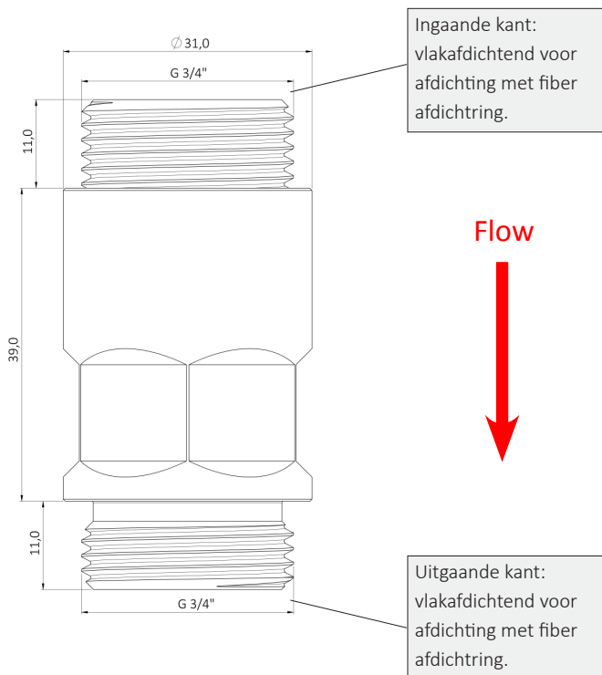
Afbeelding: HL2024 Inline 1P 3/4" (afmetingen in mm)
