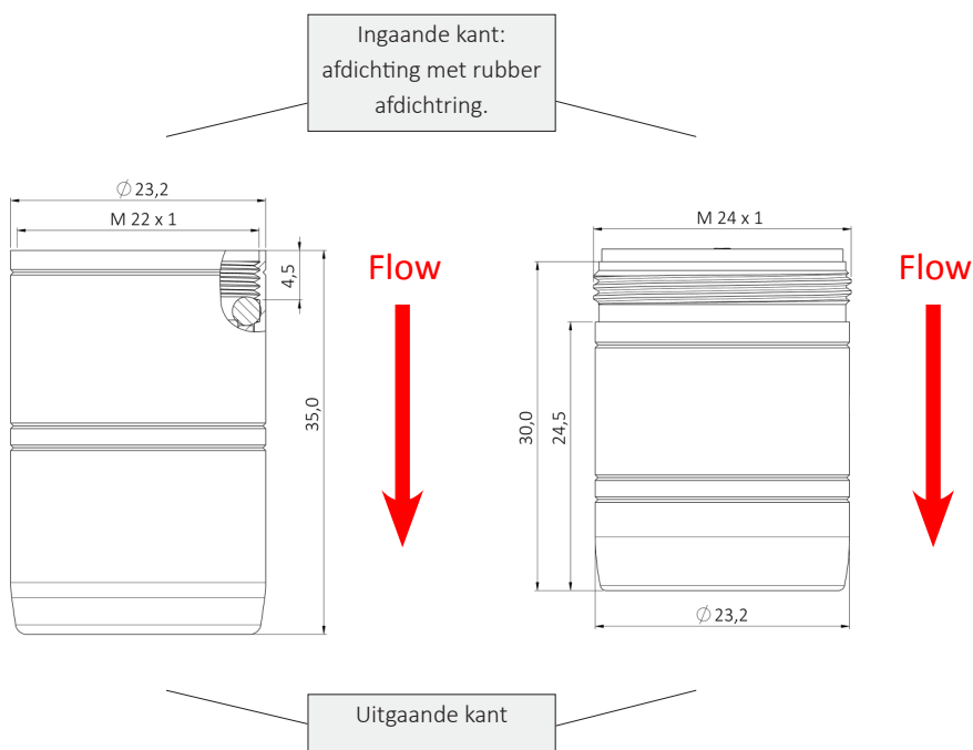
Afbeelding: HL2024 Tap M22 (afmetingen in mm)
